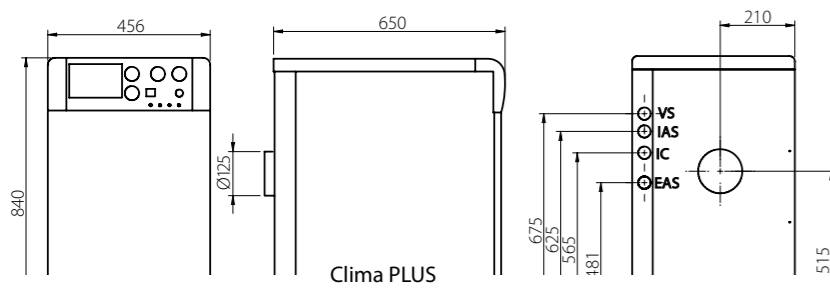
Clima PLUS
